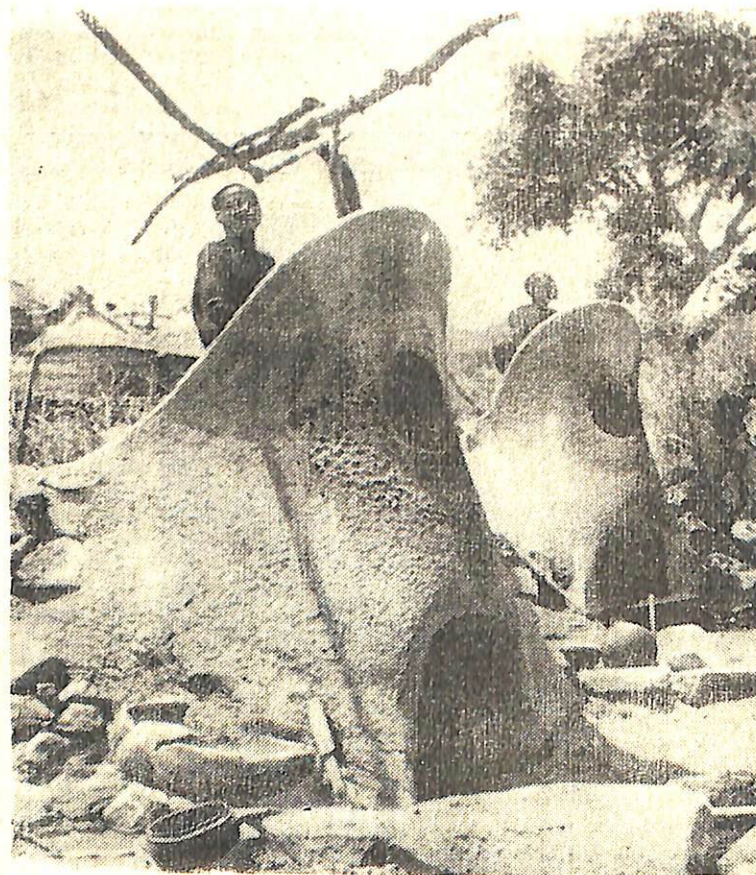
Примитивные металлургические печи племени теба в горах Мандара (Камерун).
