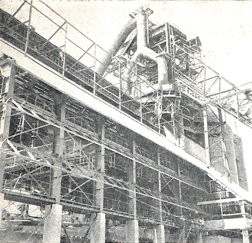
Новая домна № 1 Уханьского металлургического комбината — одна из крупнейших в Китае. По многим технико-экономическим показателям она превосходит чужейшие достижения доменного производства Англии и США.
